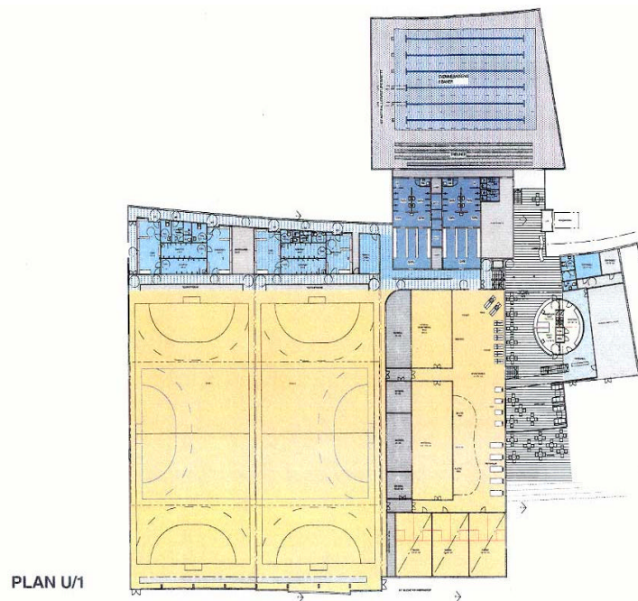
PLAN U/1 TRØNDERHALLEN MED SVØMMEHALLEN RØSTAD – ALT.1
